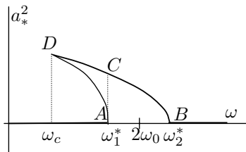
Рис. 5. Графики стационарных резонансных амплитуд в зависимости от частоты возбуждения \omega в системе с диссипацией энергии ( b > 0 ) Рис. 6. Графики стационарных резонансных амплитуд в зависимости от частоты возбуждения \omega в системе без диссипации энергии ( b = 0 )
