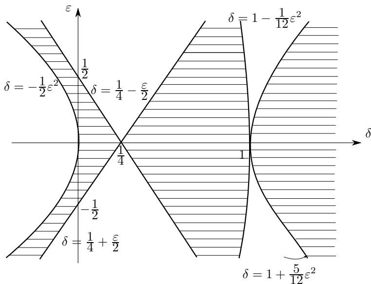
Рис. 3. Диаграмма устойчивости на плоскости параметров (\delta, \epsilon)
