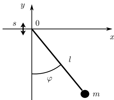
Рис. 1. Плоский математический маятник с колеблющейся точкой подвеса
