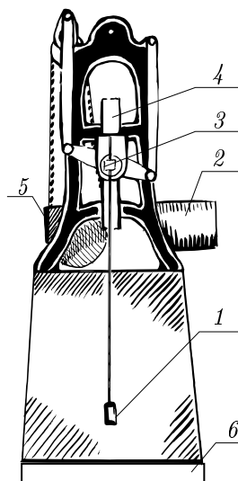
Рис. 7. Схема установки «Параметрический резонанс»
